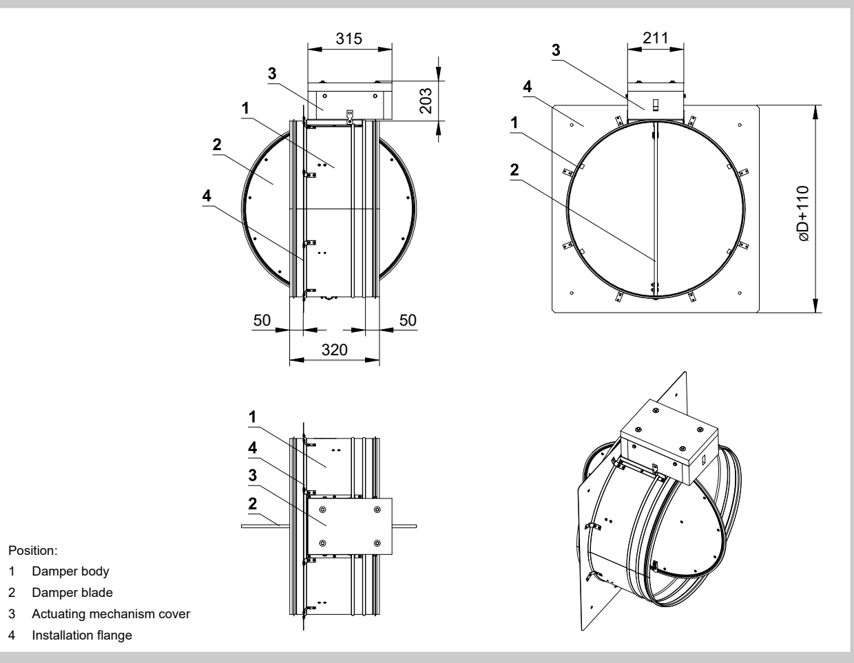
Fig. 6 Damper SEDS-R
